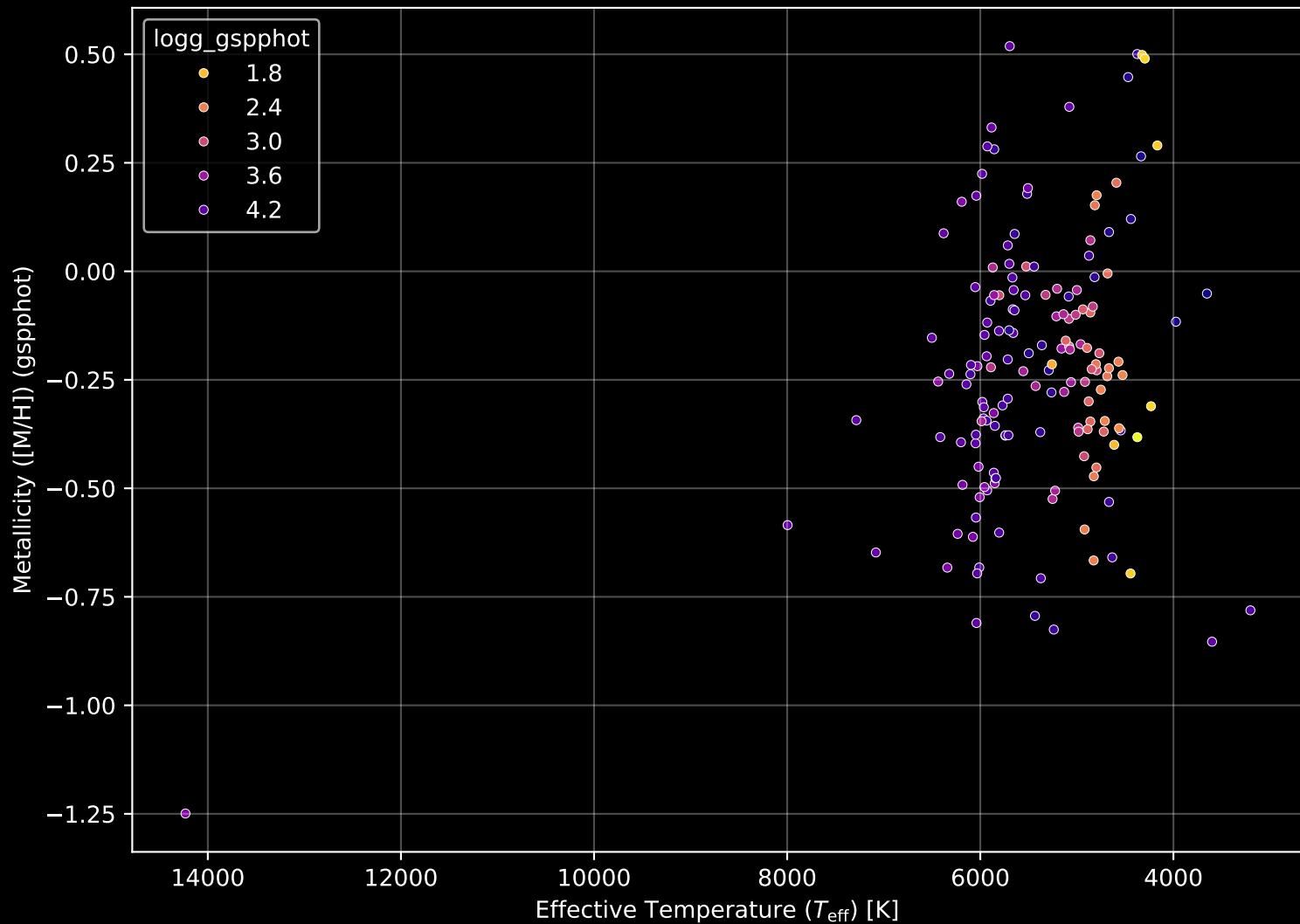
APOGEE DR17 Field: [276-28-O_TESS] Stellar Population Parameters (n= 159)
